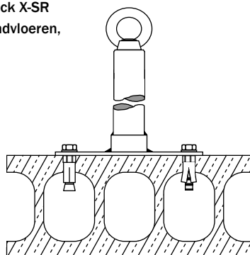
Detail ABS-Lock X DURCH t.b.v. doorsteken, incl. contraplaat
