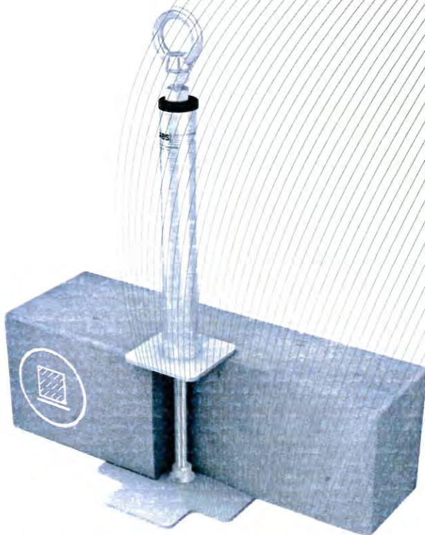
Bild 1: Anschlageinrichtung, Typ: ABS-Lock® X-DURCH (Montagebeispiel)
