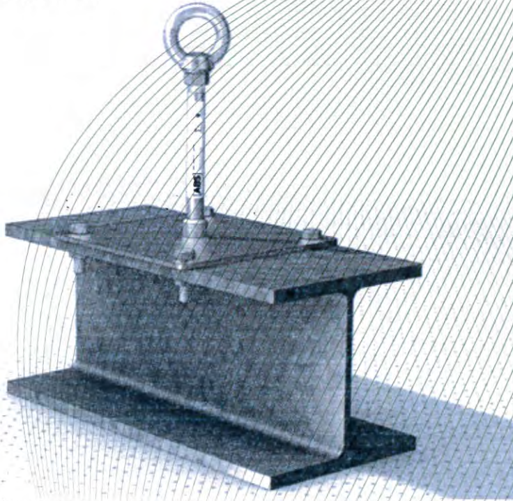
Bild 1: Anschlageinrichtung, Typ: ABS-Lock® X-ST
